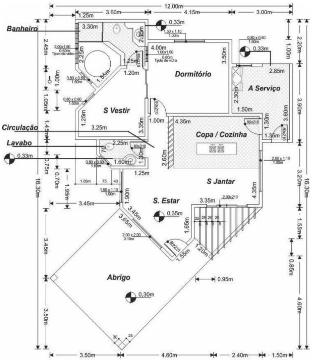
Planta Baixa - Técnica
