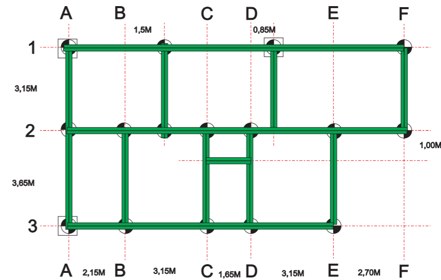
Planta de Locação
