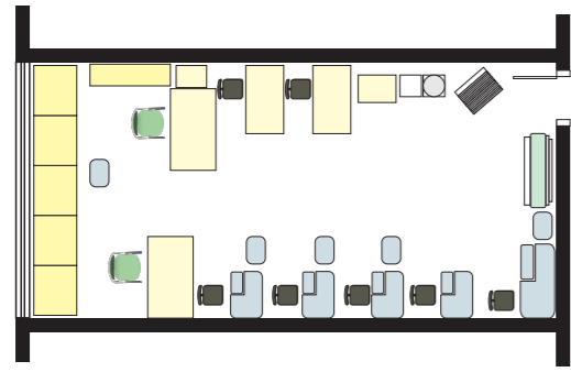
Planta baixa - sala de aula (reforma)
