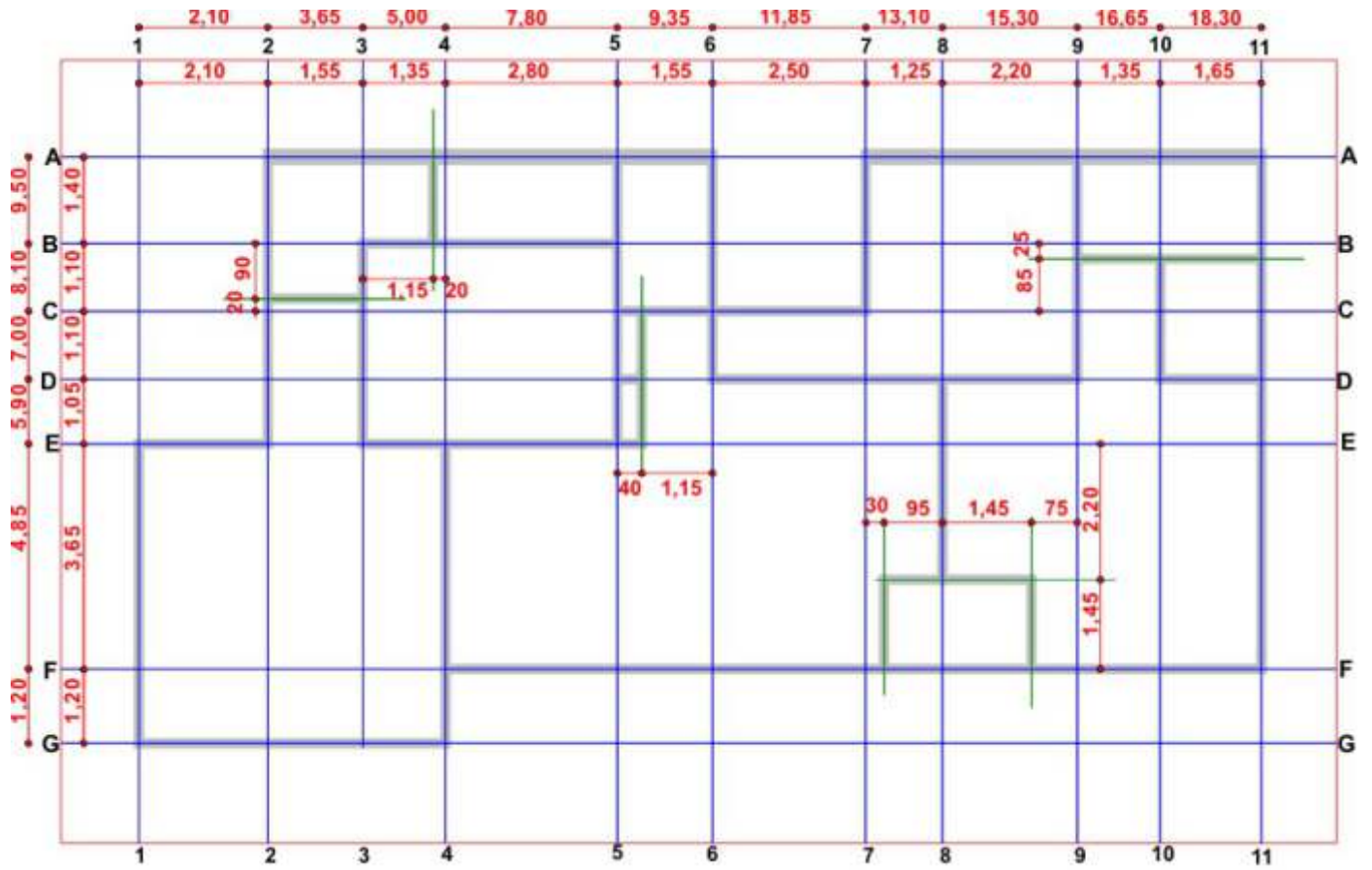
Planta - Locação de eixos
