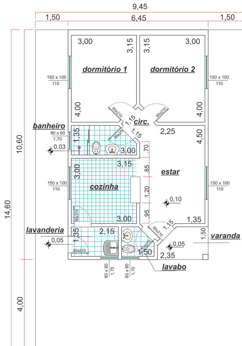
Planta baixa - técnica
