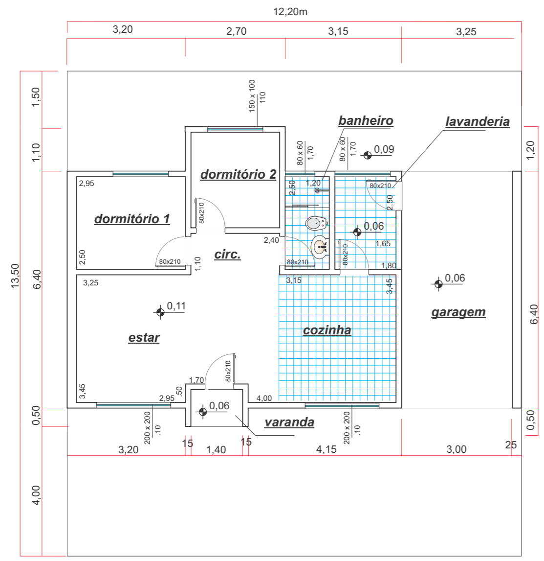
Planta baixa - técnica Escala - 1/100
