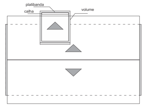
Planta de Cobertura Escala - 1/200 projeção do beiral = 0,75m
