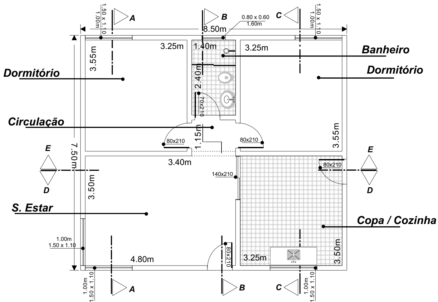
Planta Baixa - Técnica
