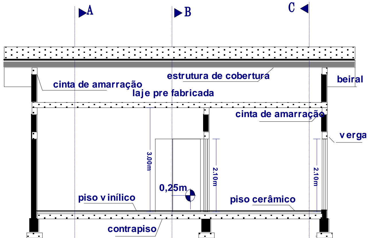
Corte EE' Escala - 1 / 50
