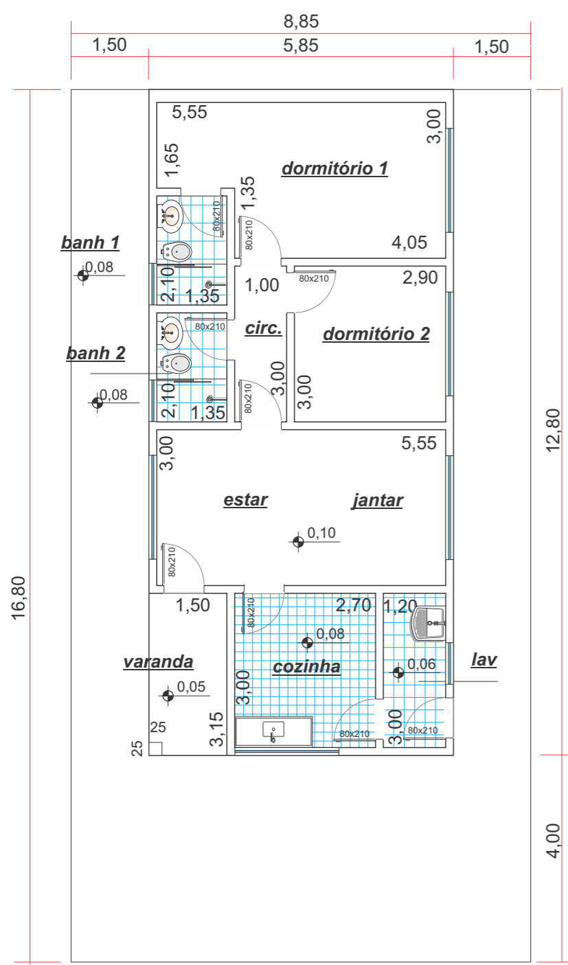
Planta baixa - técnica Escala - 1/100
