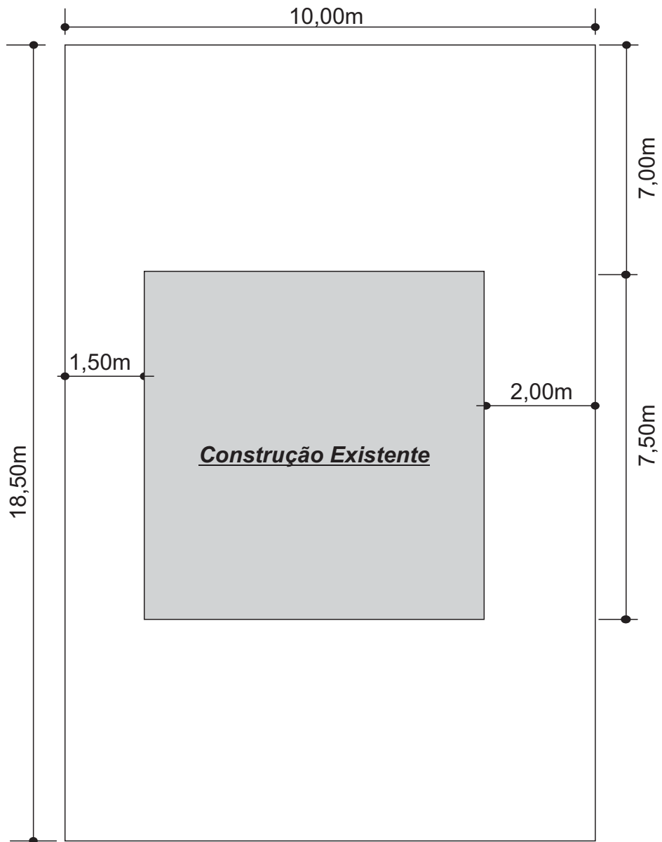
Levantamento - Terreno
